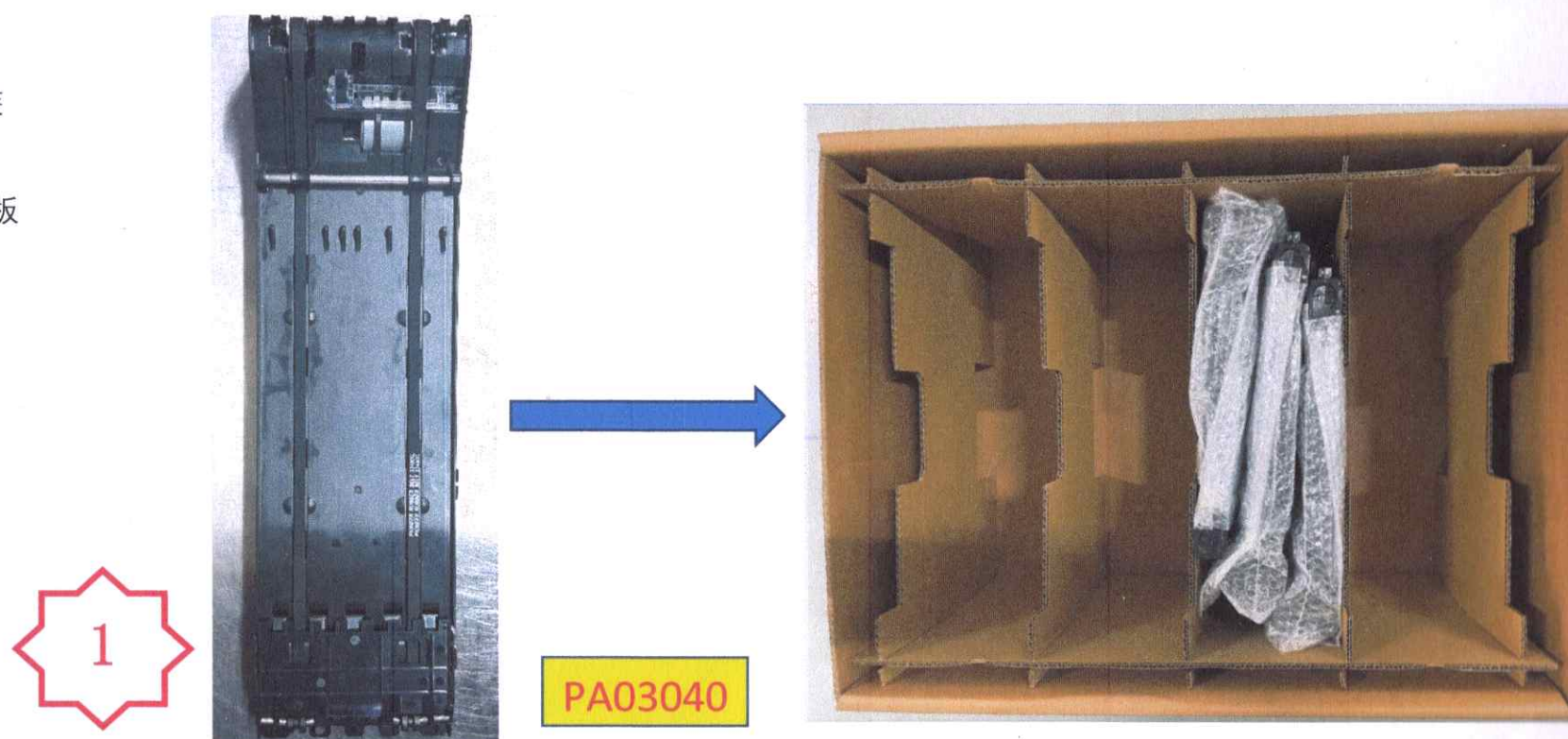
图一，每箱 4 格，每格两层，每层放 3 个中间用珍珠棉隔开，共 6 个，一箱装 24 个，确认 PA03040 组件正确装好气泡袋装入箱子（如图示）。
